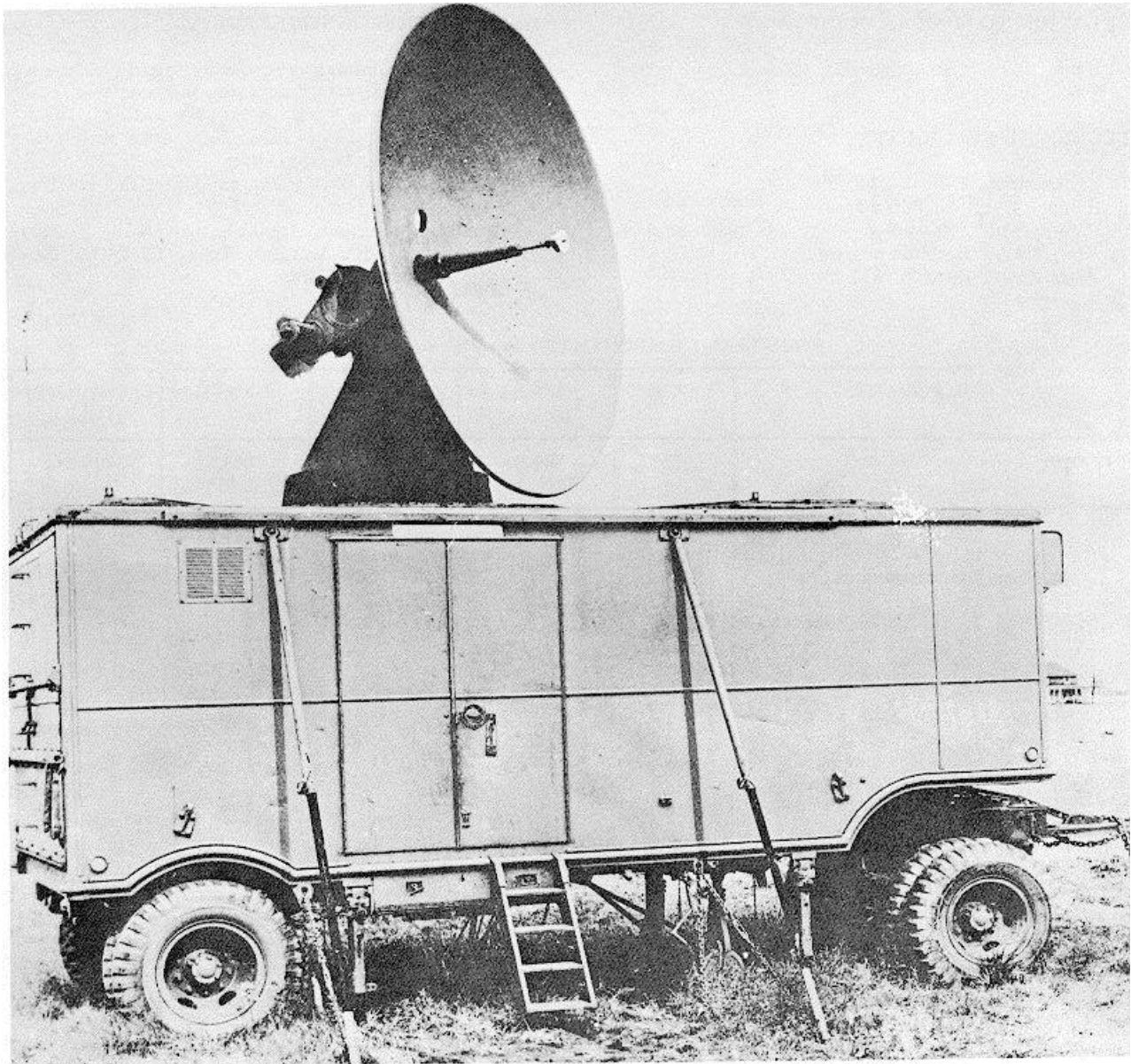
AN/MPQ-22: 1
