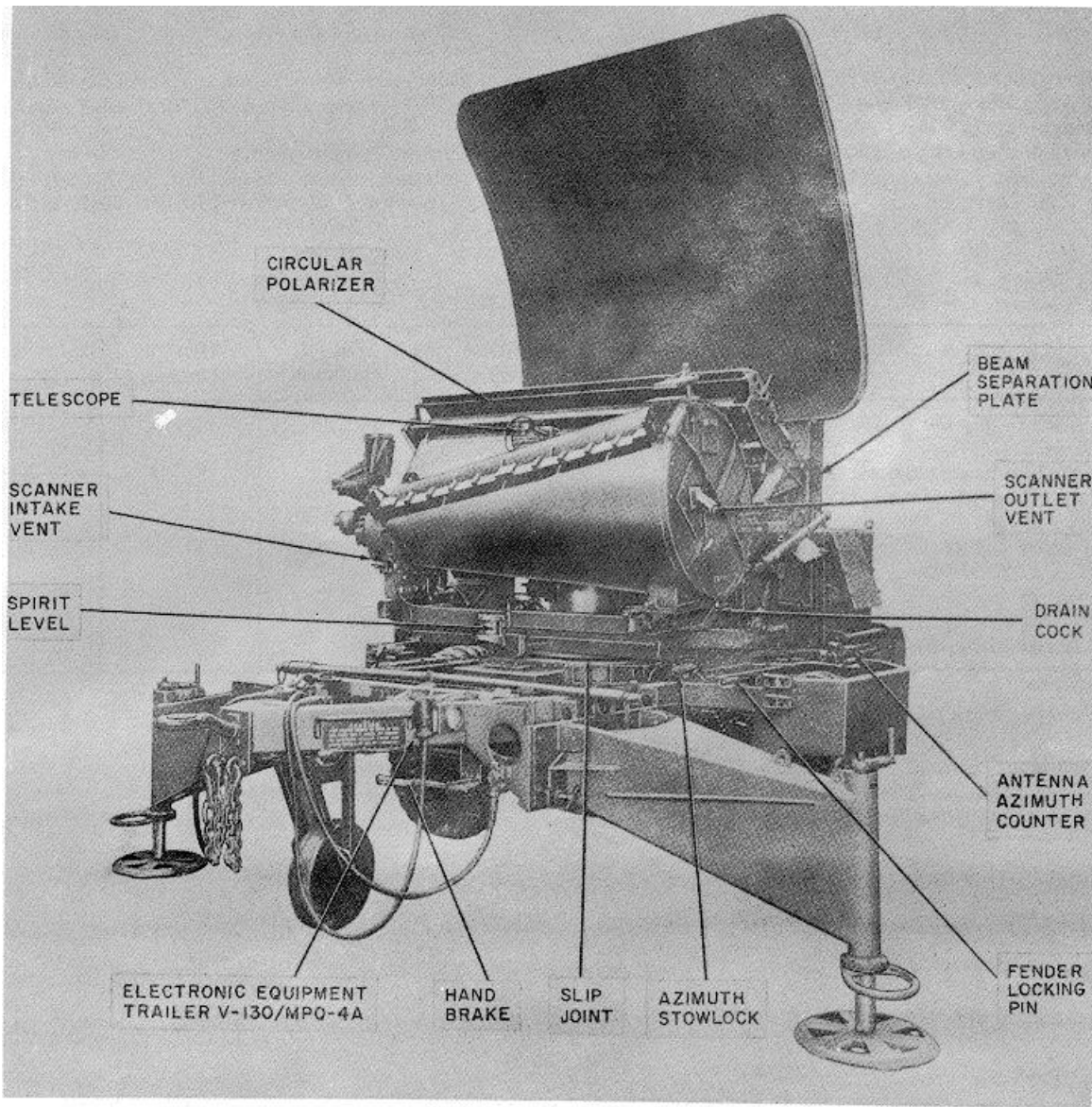
AN/MPQ-4A: 1
