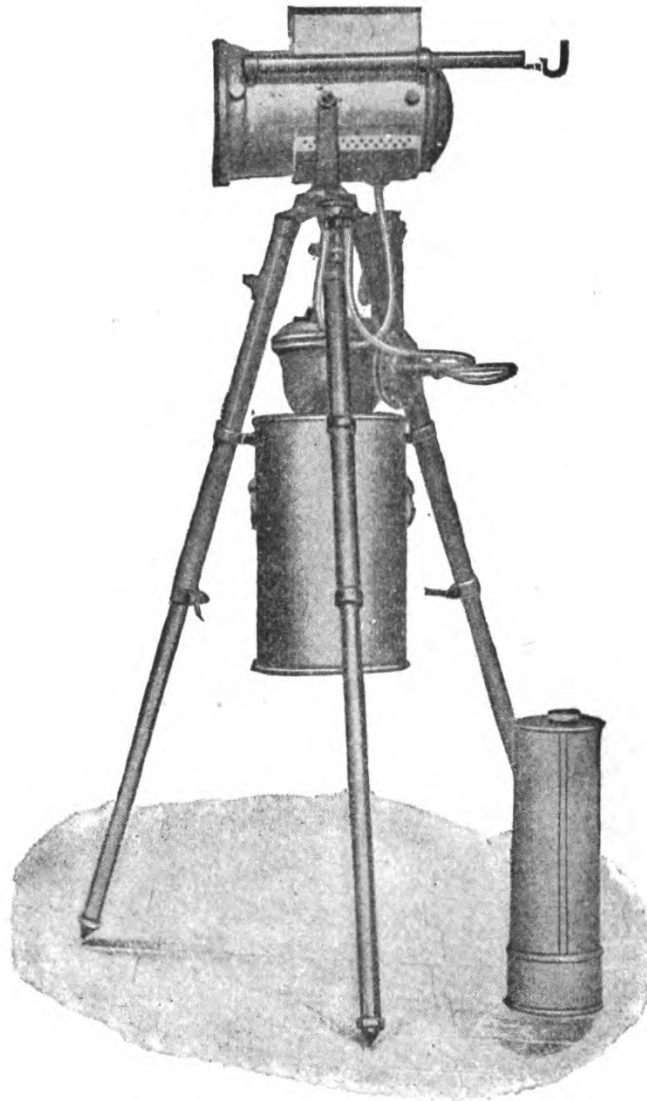
FIG. 27—Station Signaling Lantern.
