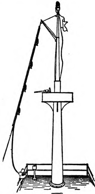
FIG. 42.—A Hoist.
