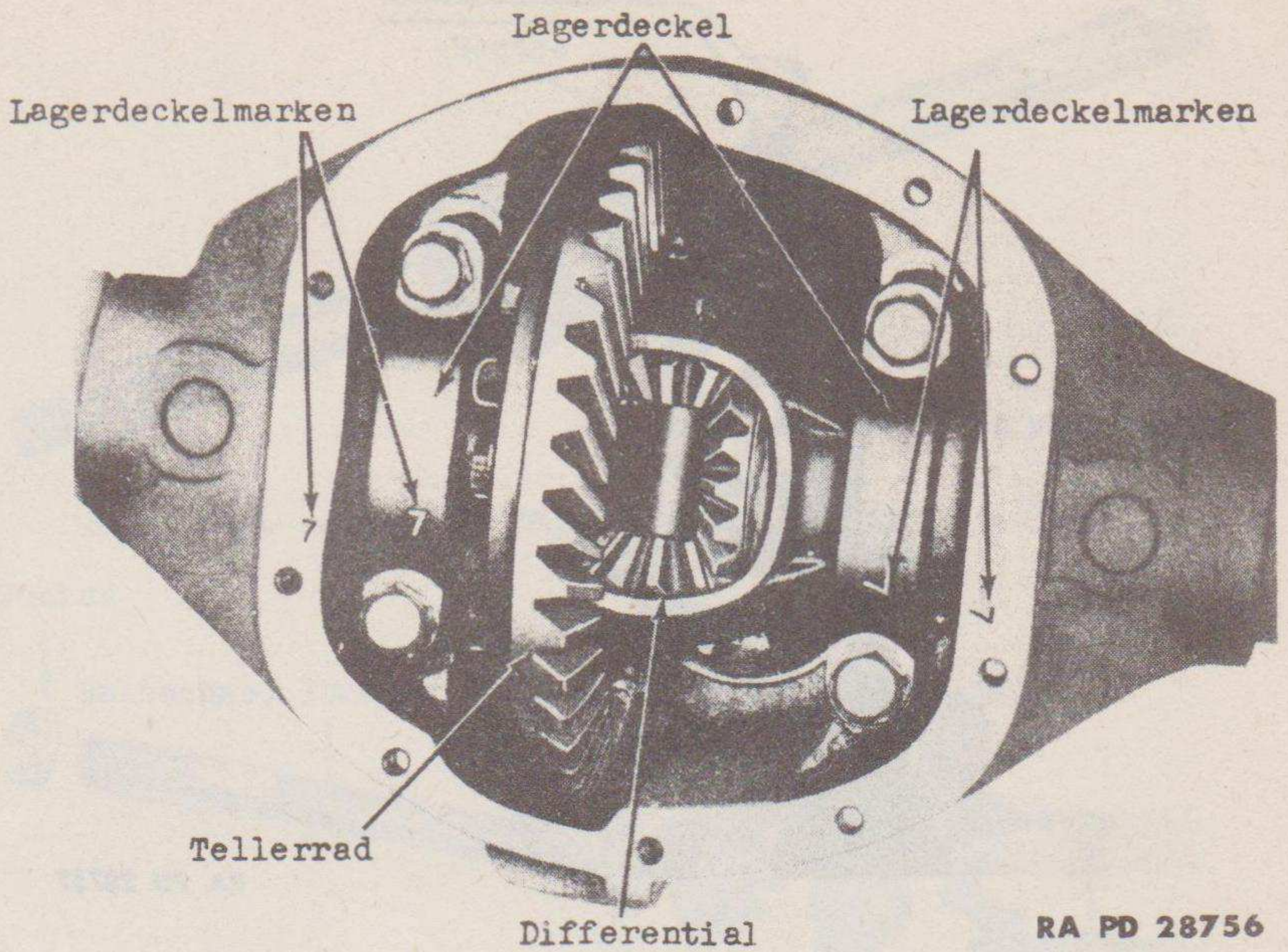
Abb. 47 - Differential-Zusammenstellung
