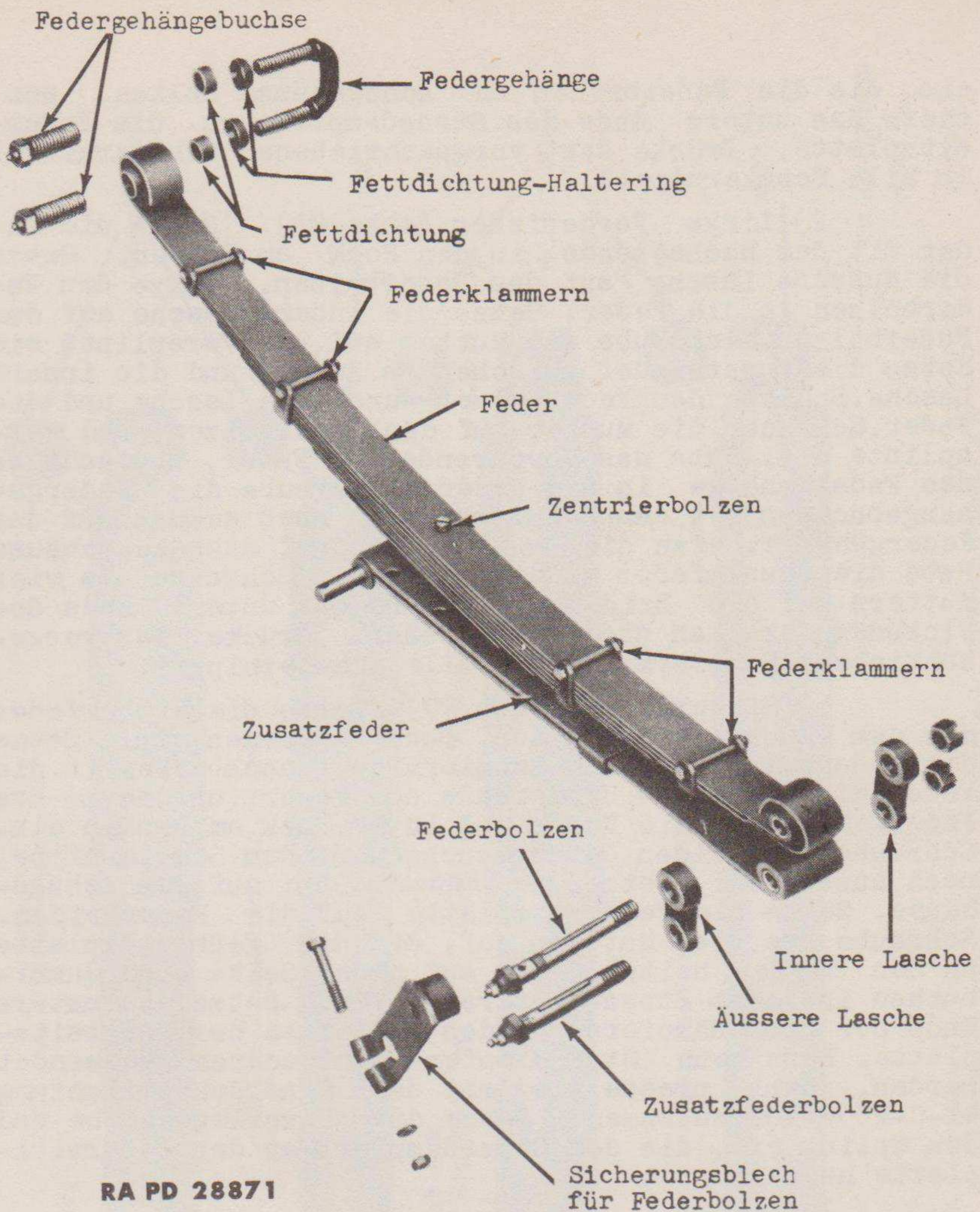
Abb. 86 - Vorderfeder - Zerlegt
