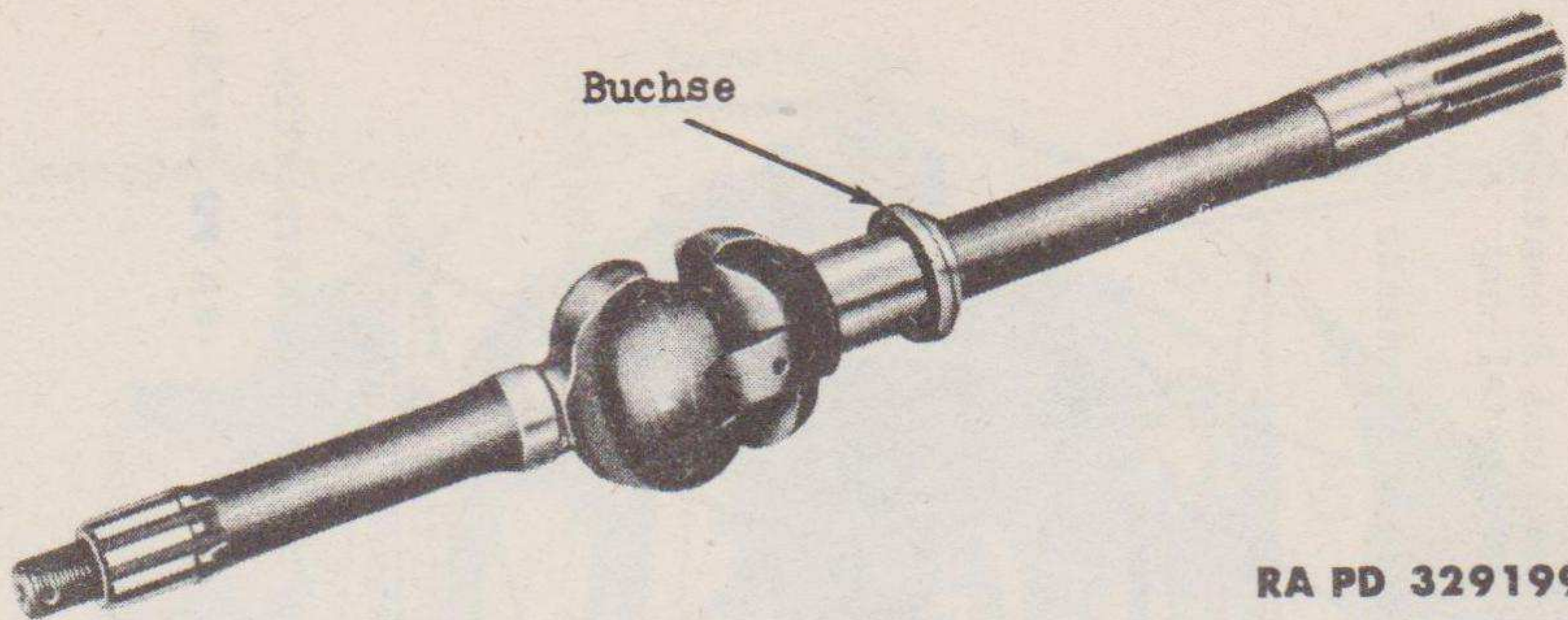
Abb. 44 - Vorderachswelle (Tracta-Typ)
