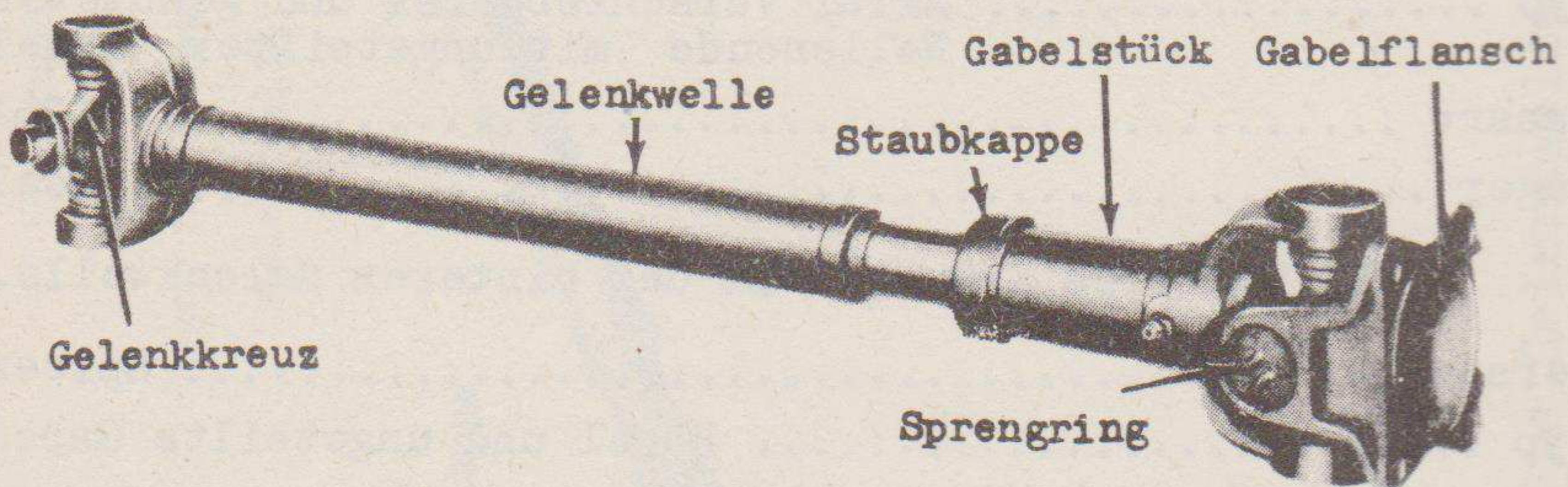
Abb. 30 - Vordere Gelenkwelle
