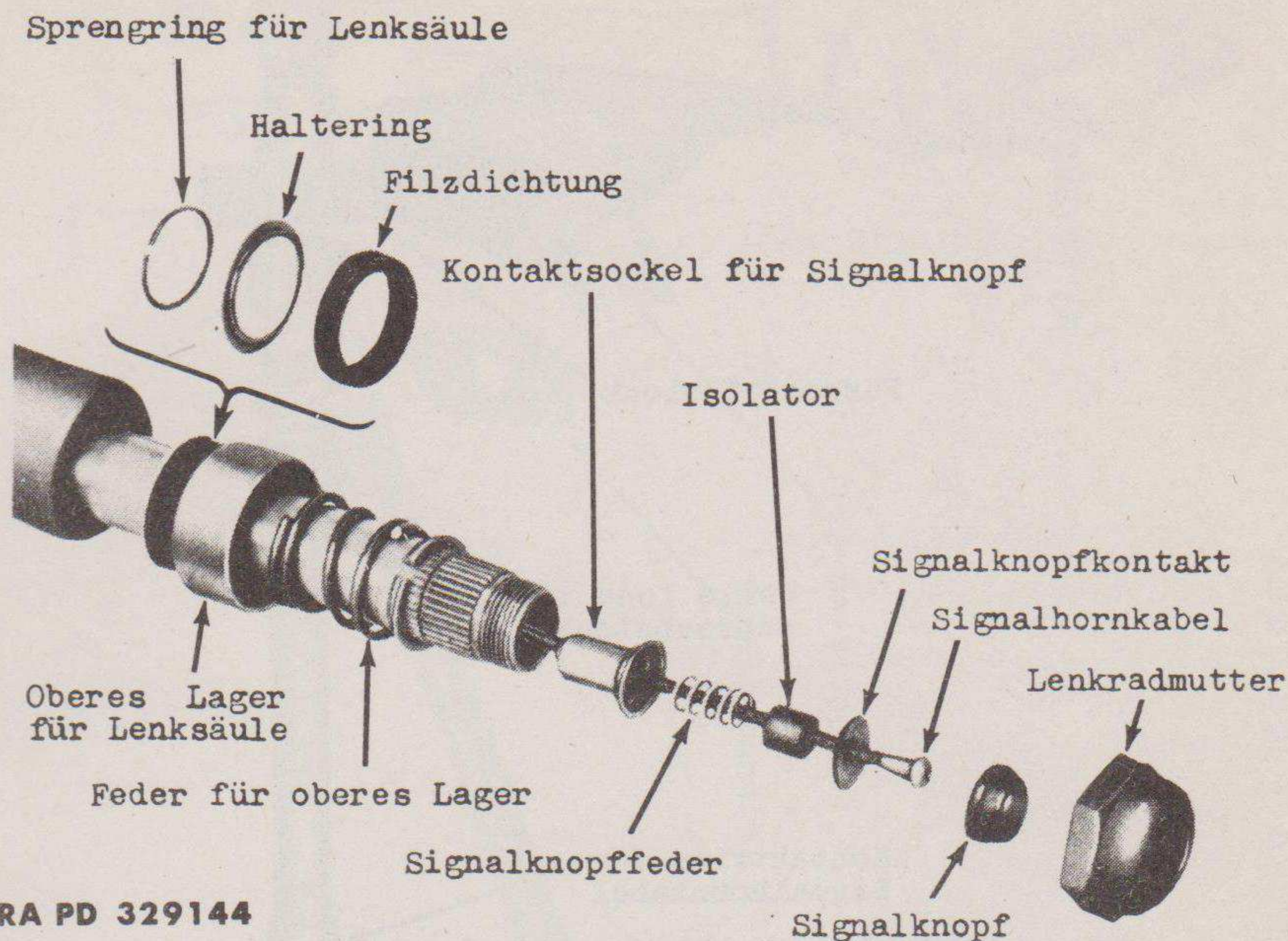
Abb. 97 - Signalknopf-Zusammenstellung - Zerlegt
